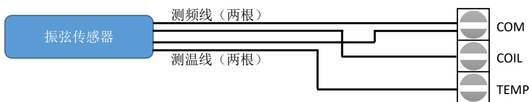
VTN208/VTN416 四线制振弦传感器连接示意图
